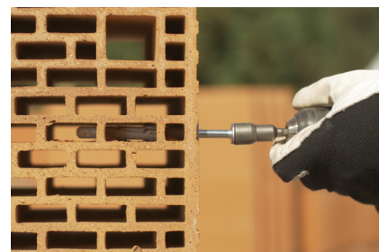
3 Закручування анкера
